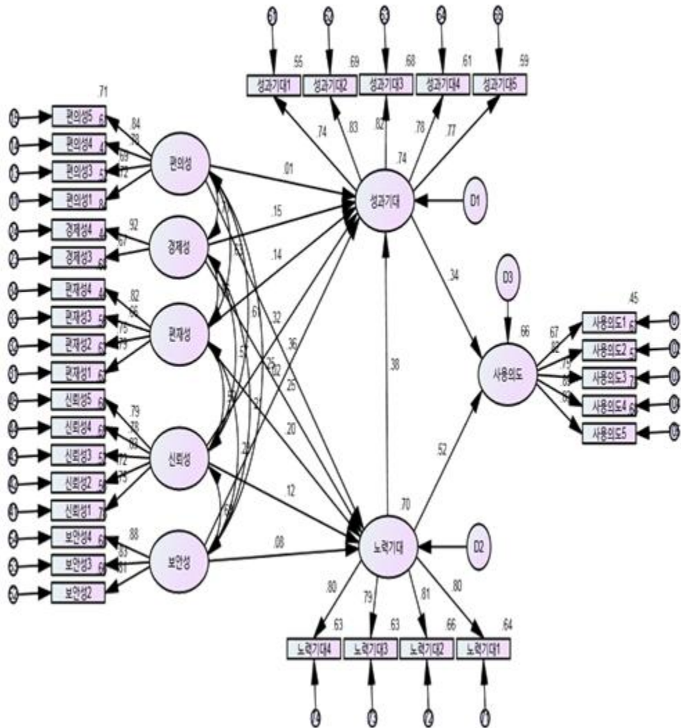
[그림 4-2] 구조방정식모델
