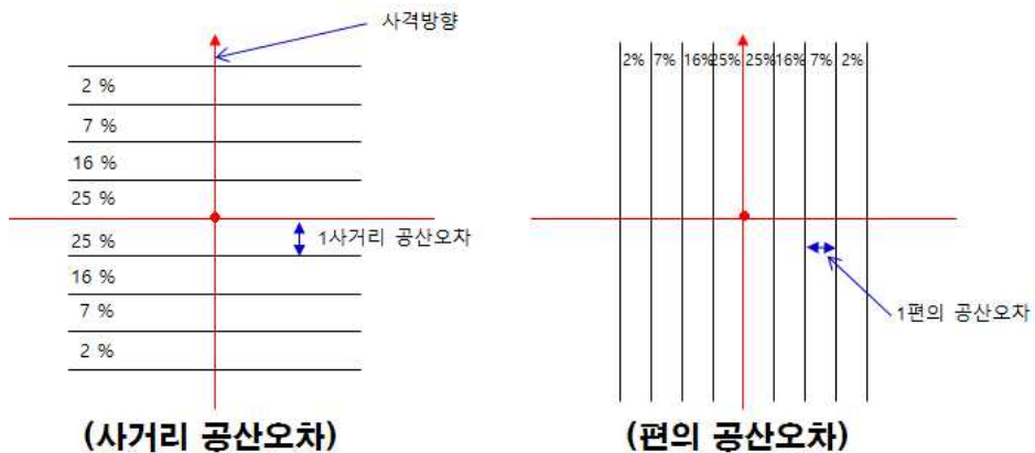
[그림 2-1] 사거리 및 편의 공산오차
