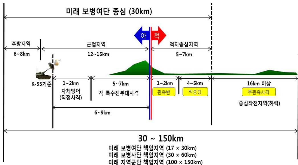
[그림 3-1] 중심지역 관측 제공
