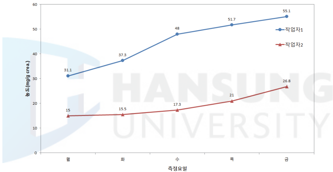
[그림 3] 요일별 삼염화초산 평균농도 변화.
