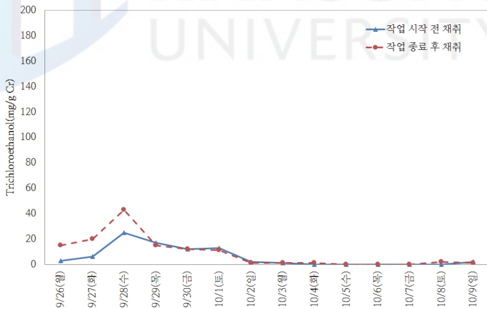
[그림 11] 작업자 2의 작업 전후 소변 중 삼염화에탄올 농도.
