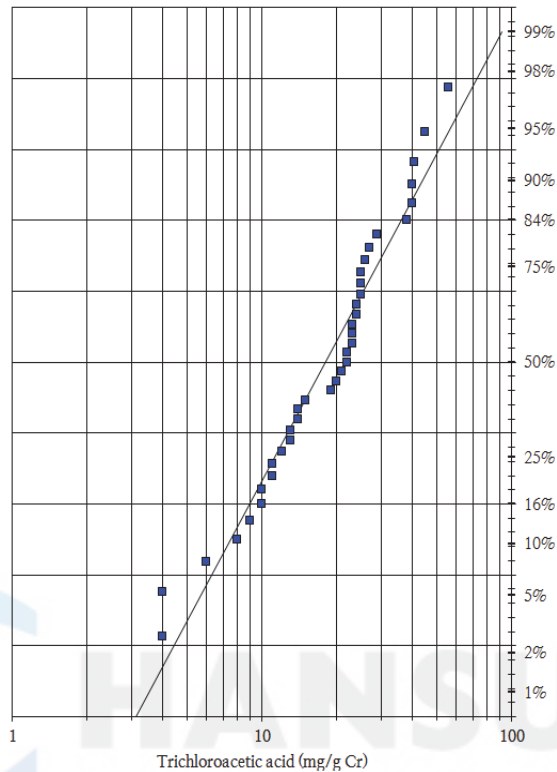
[그림 7] 작업자 2의 소변 중 삼염화초산 농도.
