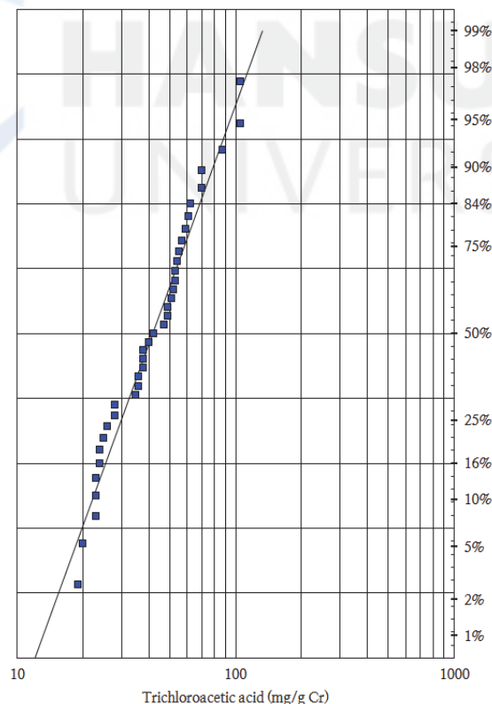
[그림 6] 작업자 1의 소변 중 삼염화초산 농도.
