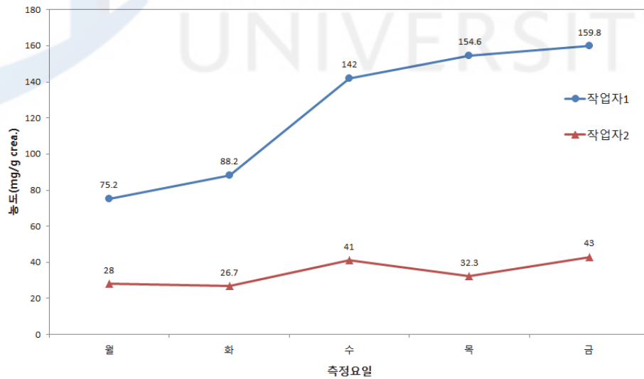
[그림 5] 요일별 총삼산화물 평균농도 변화.
