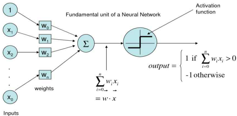
[그림 2-14] 퍼셉트론(Perceptron) 구조
