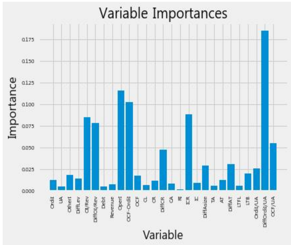
[그림 4-7] Random Forest를 이용한 2016년 예측모델의 변수 중요도
