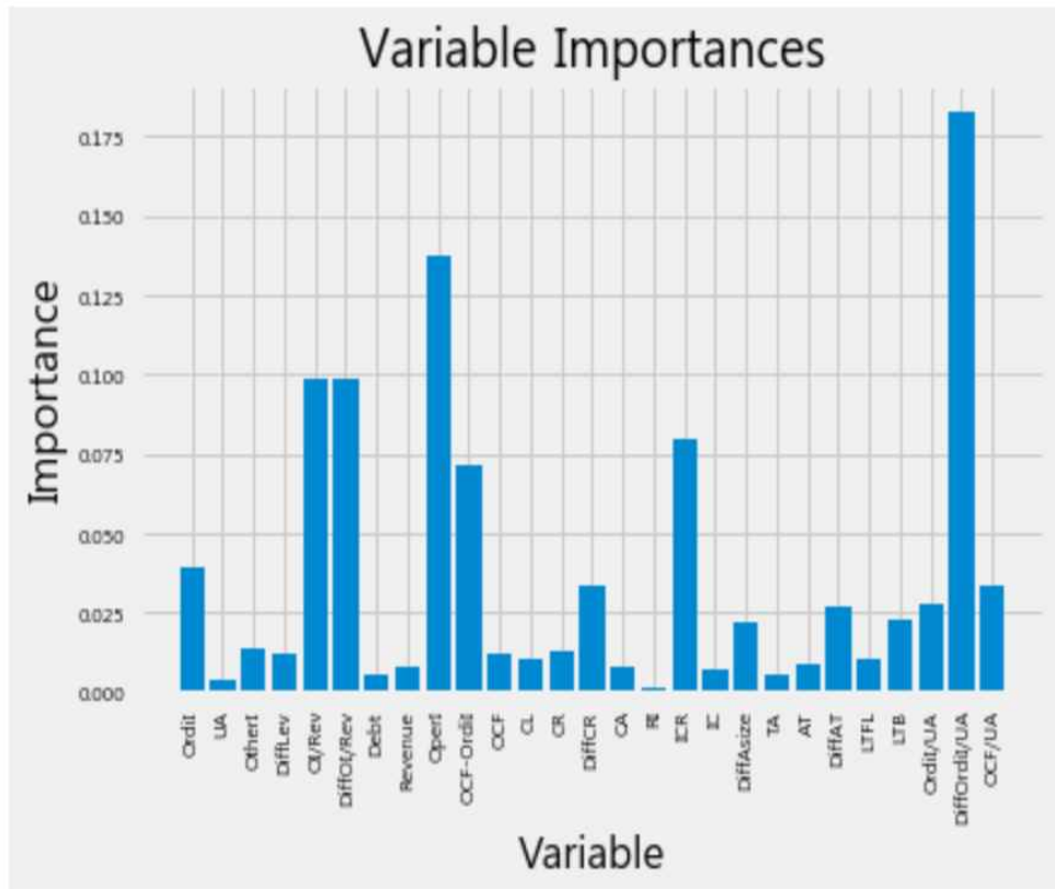
[그림 4-8] Random Forest를 이용한 2017년 예측모델의 변수 중요도
