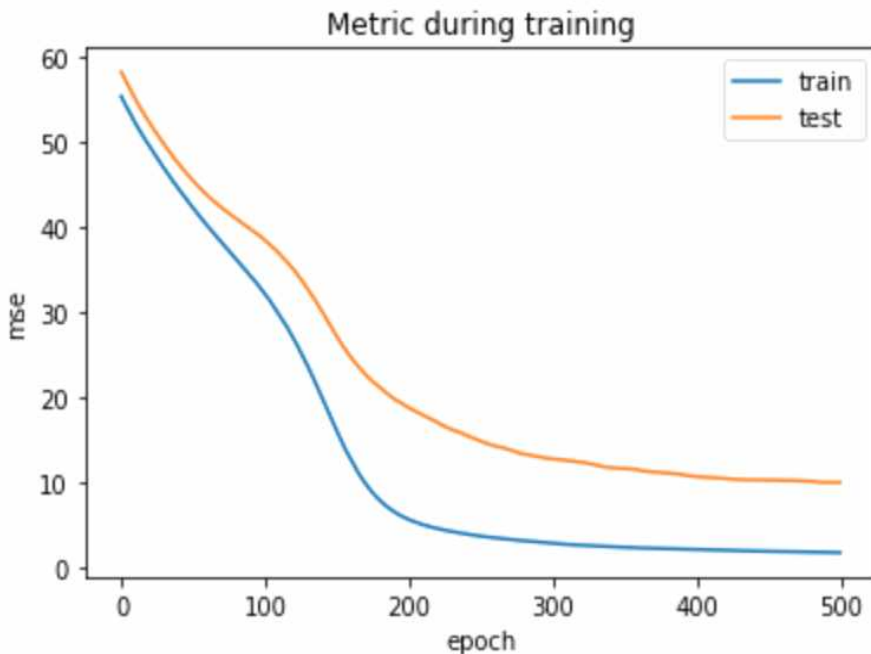
[그림 4-15] DNN을 이용한 2016년 예측모델의 epoch에 따른 MSE
