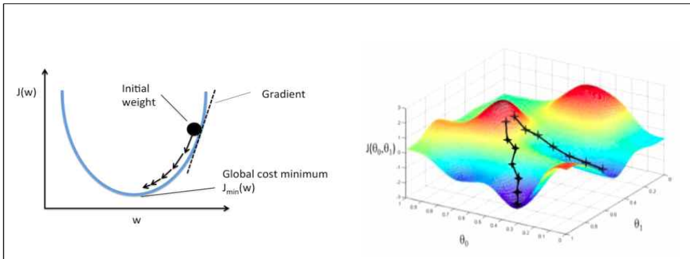
[그림 2-18] 경사하강법(Gradient Descent) 개념도
