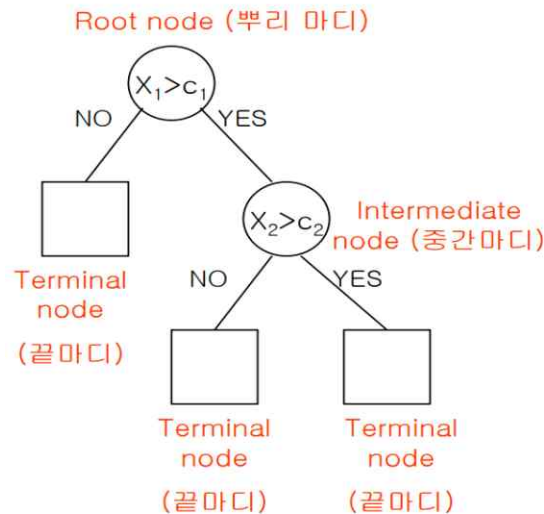
[그림 2-5] 의사결정트리의 구성요소
