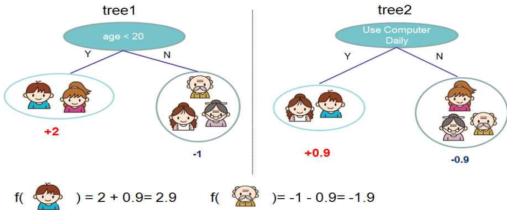
[그림 2-9] 트리 앙상블 모델의 최종 결정값 계산
