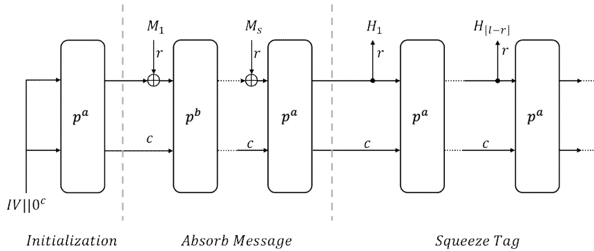
[그림 2-2] ASCON 해시함수 암호화 과정
